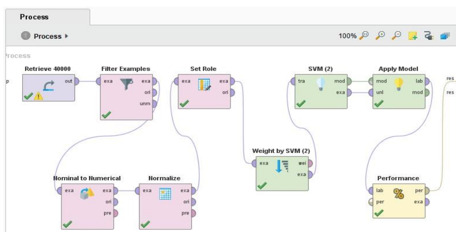
شکل ۵: پیاده‌سازی الگوریتم ماشین‌بردار پشتیبان در ریپدماینر
