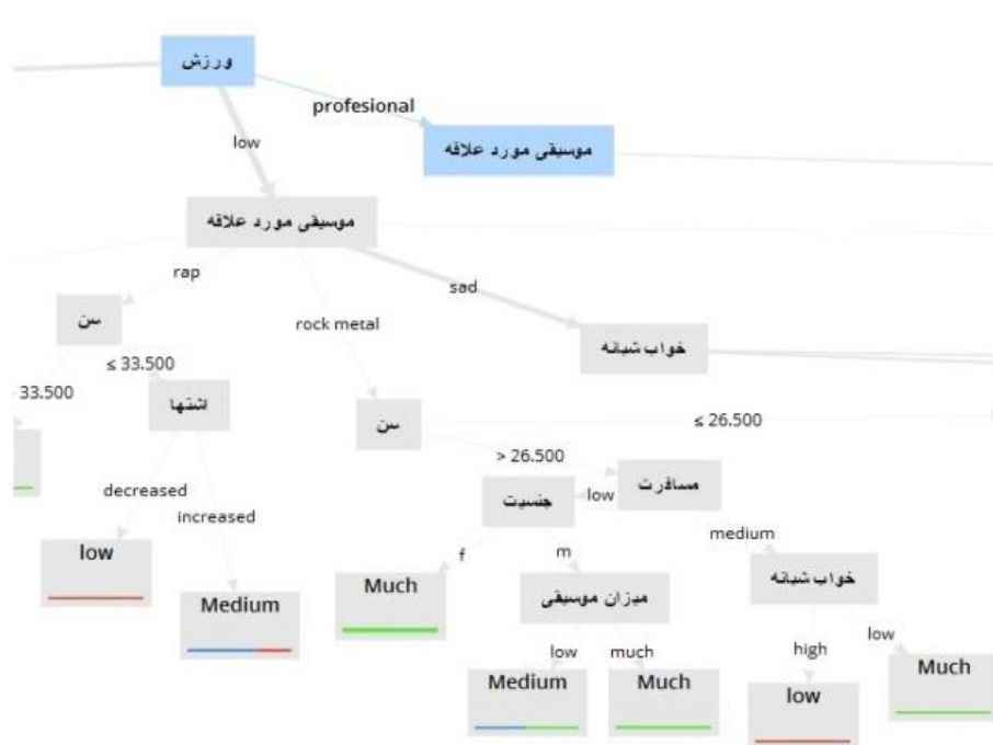
شکل ۱: بخشی از نتیجه درخت تصمیم در پیدماینر
